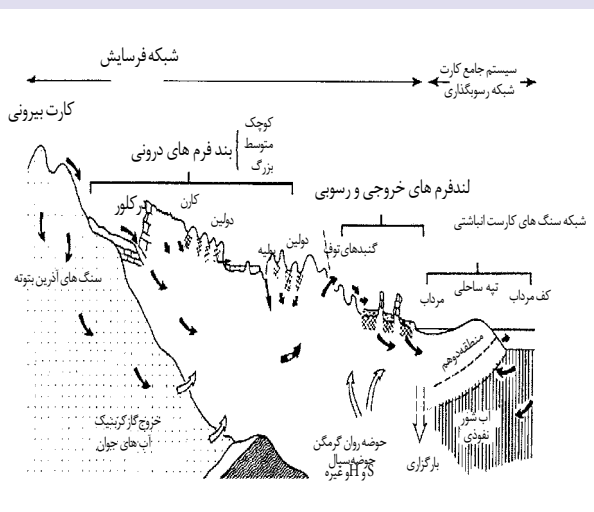
شکل ۲. سیستم جامع کارست. جوان سوئیچ، لندفرم‌های بخش ورودی، چرخه آب جوی در درون زمین و فرسایش ساحل آدریاتیک را بررسی کرد. امروزه در کارهای علمی و مهندسی، کلمه کارست کاربرد گسترده‌ای دارد.
