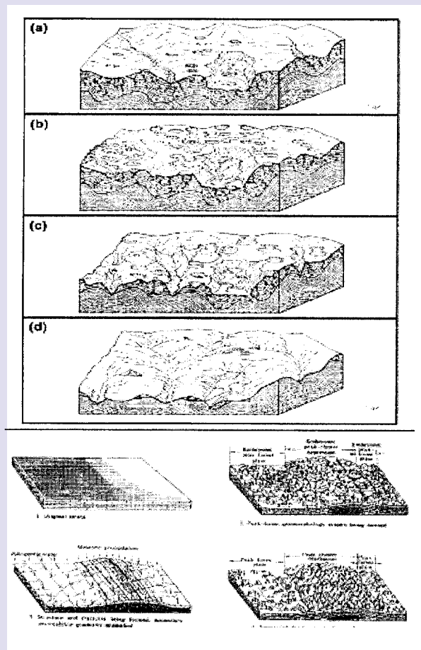
شکل ۵. مدل چرخه فرسایش در منطقه کارست براساس مدل جووان سویچ (۱۹۱۸)، تصویر بالا). مدل توسعه لندفرم‌های کارست در منطقه گویلان گوانگ‌زی چین براساس مدل زائو (۱۹۸۸)، تصویر پایین).
