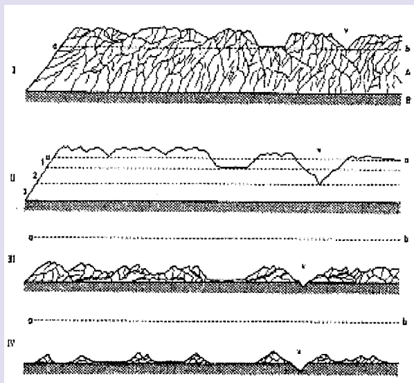
شکل ۴. تکامل تدریجی چرخهٔ آب زیرزمینی و توسعهٔ ناهمواری کارست مدل سویچ (۱۹۱۸) پس از اصلاحاتی به‌دست رولیک (۱۹۷۲).
